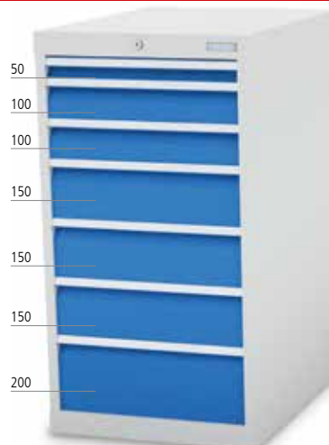
■ 7 x Schublade
