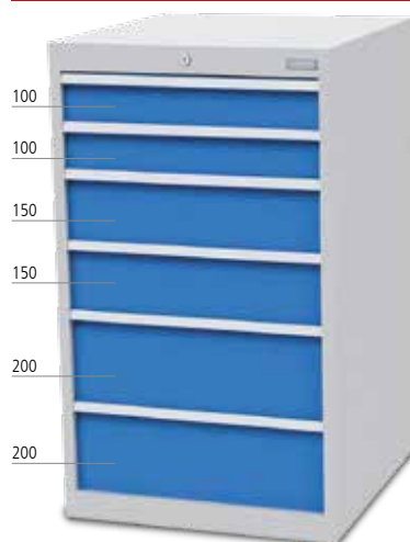
■ 6 x Schublade
