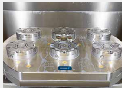
Die VERO-S Spannstation ist eine Präzisionschnittstelle zum Maschinentisch und ermöglicht das schnelle Rüsten jeglicher Spannelemente.
